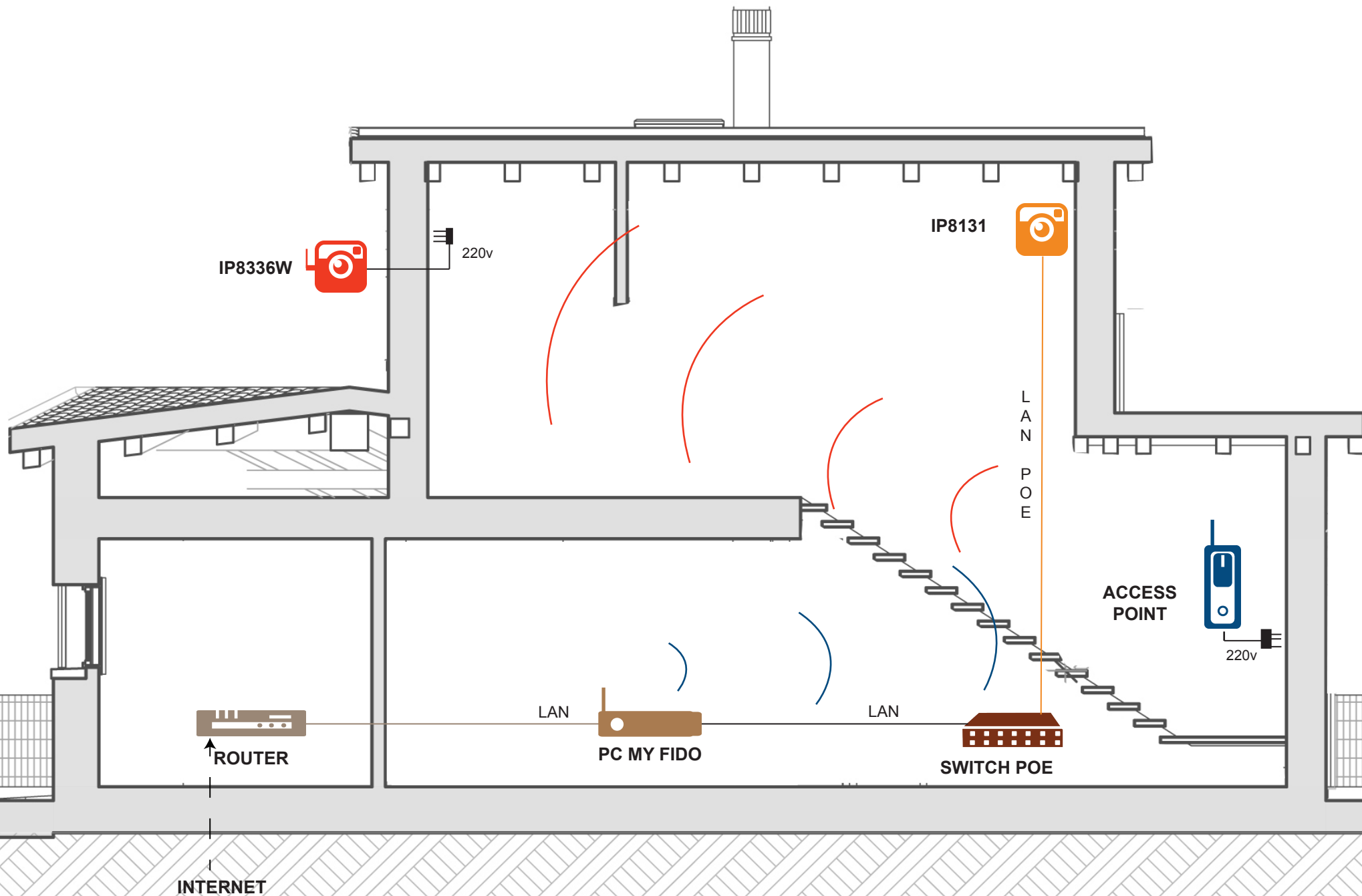
MY FIDO CLOUD MISTO WI FI - LAN
